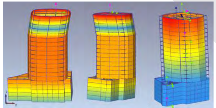
Modos de vibrar identificados con técnicas de análisis modal operacional
