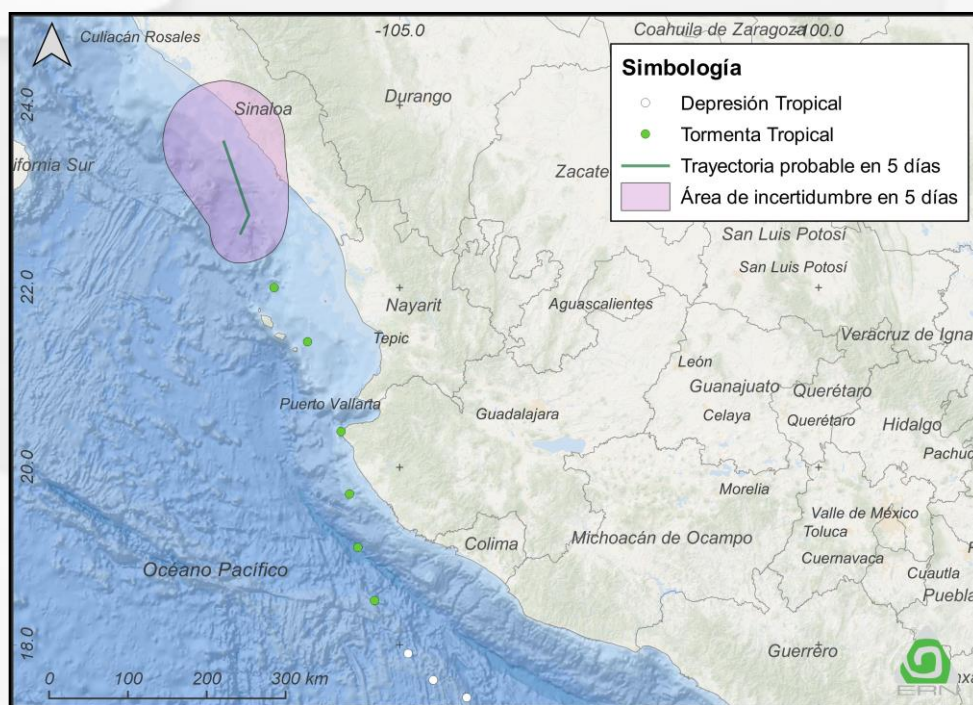
Trayectoria parcial y pronóstico para cinco días de la Tormenta Tropical Pilar. Fuente: NHC-NOAA Partial path and five-day forecast of Tropical Storm Pilar. Source: NHC-NOAA
