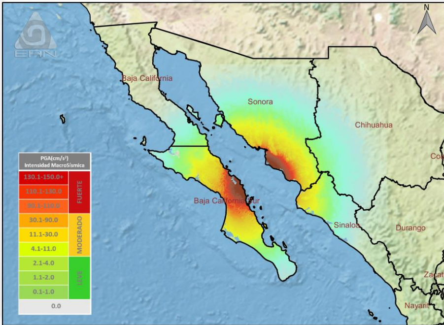
Mapa de aceleración máxima del suelo Peak ground acceleration map
