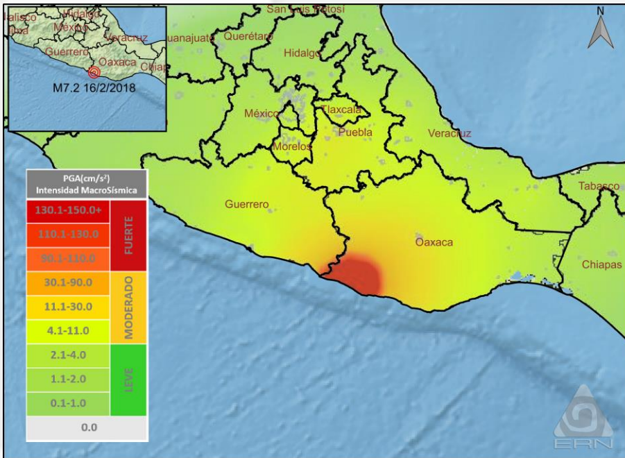
Mapa de aceleración máxima del suelo, elaborado de forma automática por el Instituto de Ingeniería, UNAM Peak ground acceleration map, elaborated automatically by the Institute of Engineering, UNAM
