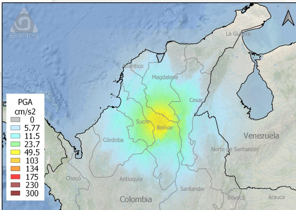
Mapa de aceleración máxima del terreno (cm/s²) / PGA map (cm/s²)
