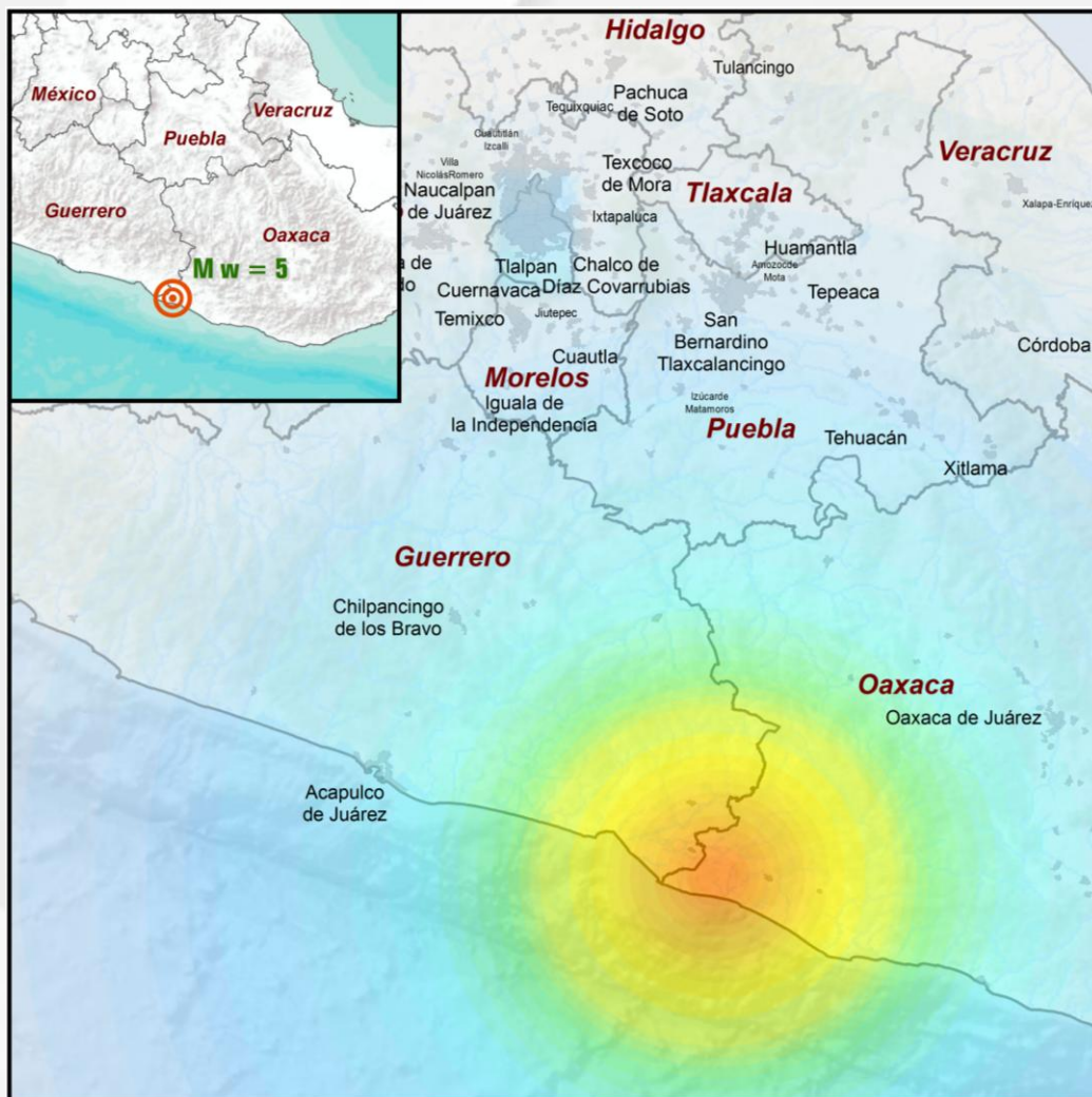
Mapa de aceleración máxima del suelo (Amax) y ubicación del epicentro del sismo de magnitud M_w = 5 con datos del SSN.
